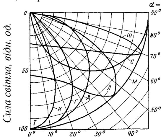
Рис. 4. Типи КСС
