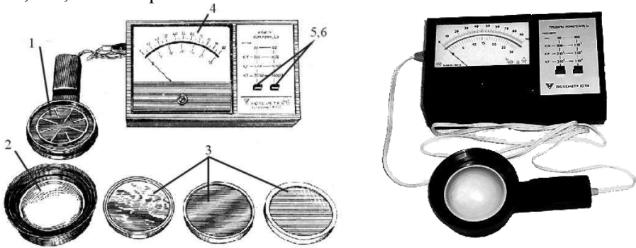
Рис. 2. Люксметр Ю-116.
