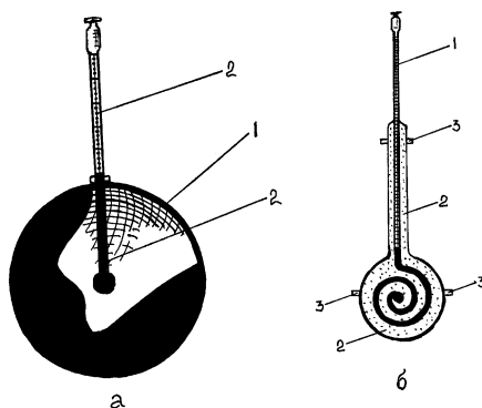
Рис. 3. Термометри для вимірювання радіаційної температури: а – Кульовий чорний термометр в розрізі (1 – куля діаметром 15 см, покрити матовою чорною фарбою; 2 – термометр з резервуаром в центрі кулі); б – Пристінний термометр з плоским спіралью вигнутим резервуаром (1 – термометр; 2 – базова обкладинка (поролон); 3 – клейка стрічка)
