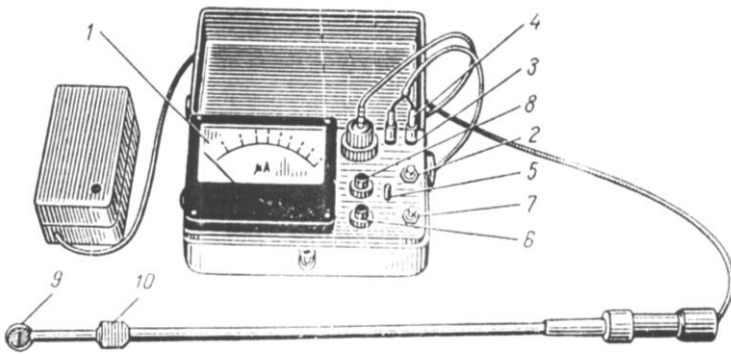
Рис. 4. Електротермоанемометр (1 – гальванометр; 2 – перемикач живлення; 3 – клеми для підключення до мережі; 4 – вилка датчика; 5 – перемикач для визначення температури або швидкості руху повітря; 6 – перемикач «вимірювання – контроль»; 7 – ручка регулювання напруги; 8 – датчик (мікро-термоопір); 9 – захисний футляр датчика.)
