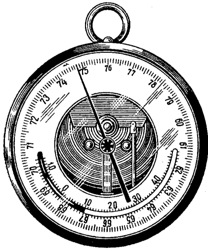
Рис. 5. Барометр-анероїд
