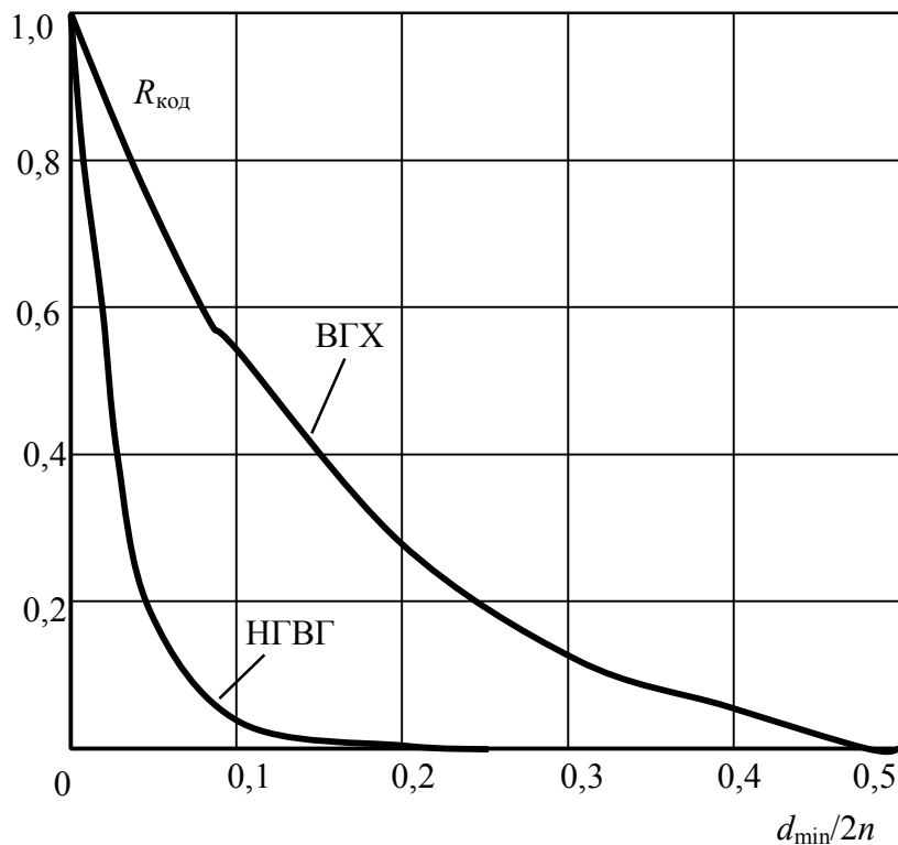
Рисунок 6.1 – Кодові границі блокових кодів
