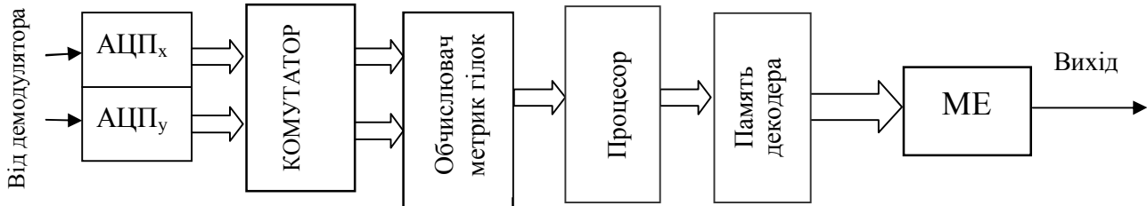
Рисунок 10.3 – Структурна схема декодера Вітербі
