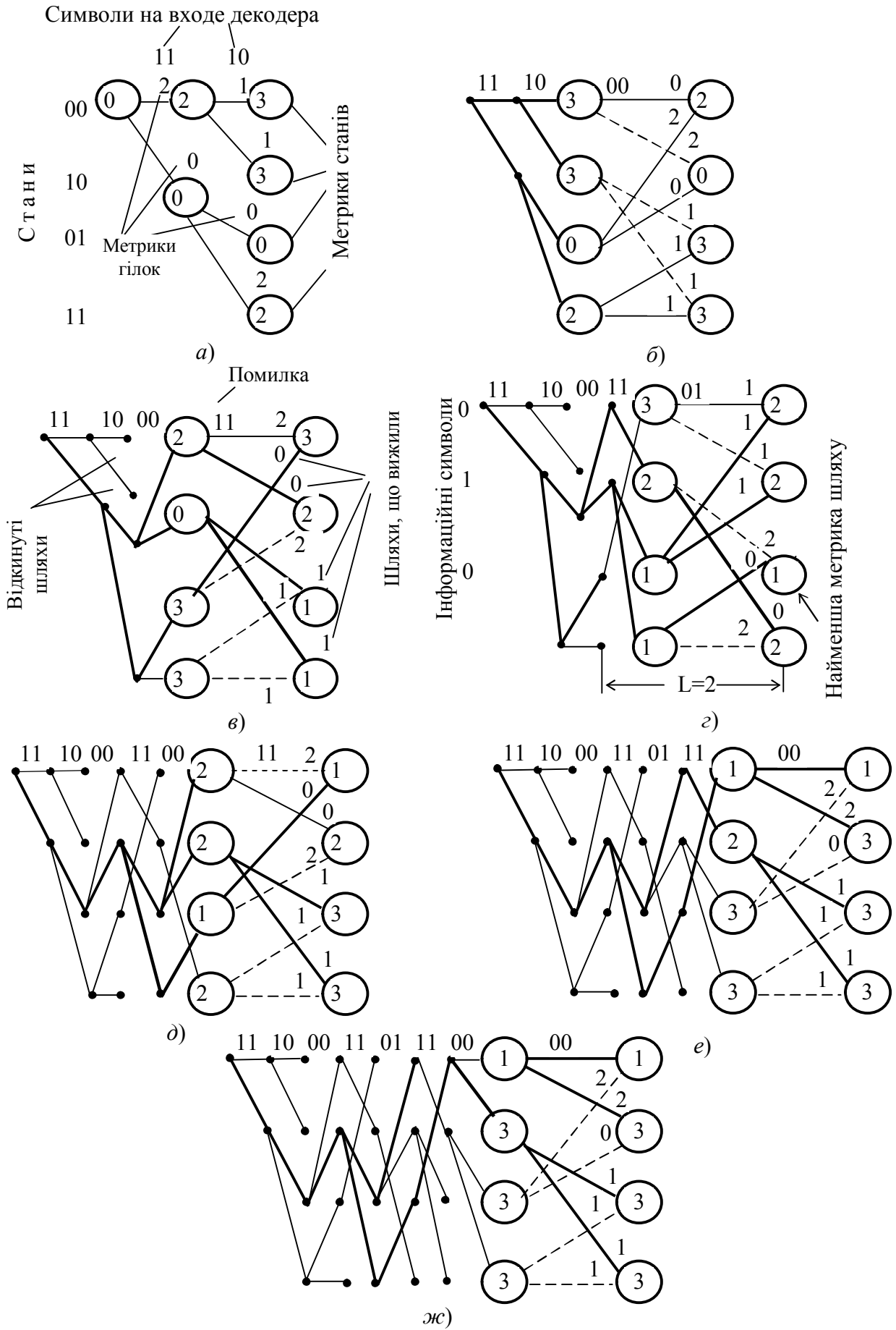
Рисунок 10.2 – Декодування коду (7,5)
