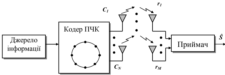
Рисунок 13.10 – Модель системи с просторово-часовим кодуванням
