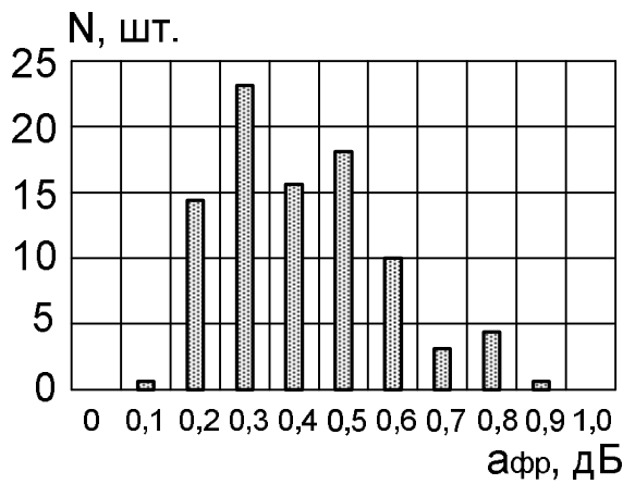
Рисунок 8.3 – Діаграми розподілу втрат в одномодових ОВ з'єднувачах HMS-10/HP: а – втрати, що вносяться, б – зворотні втрати
