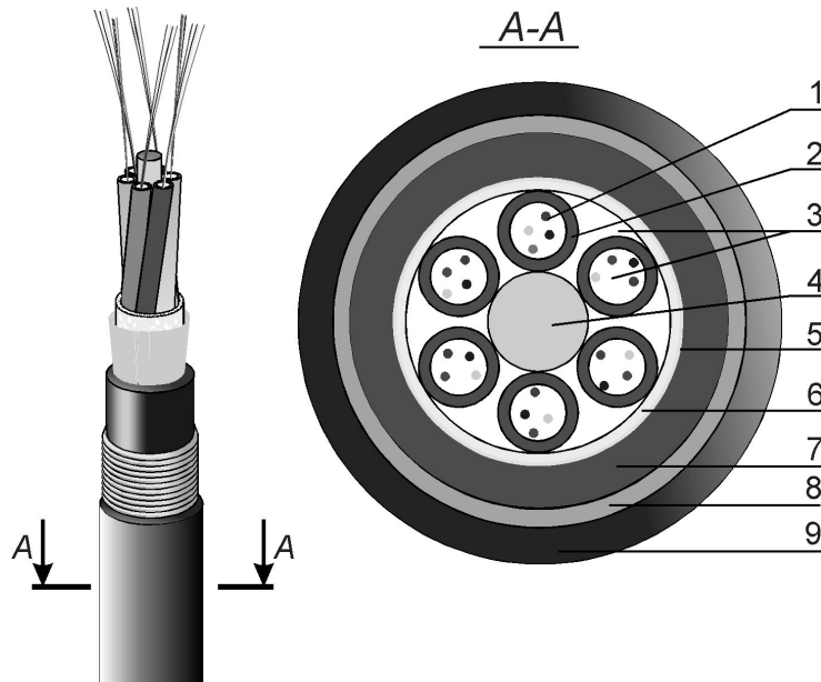
Рисунок 11.3 – Самонесучий ОК модульної конструкції зі сталеву гофрованою оболонкою (MASS): 1 – ОВ; 2 – оболонка оптичного модулю; 3 – гідрофобний заповнювач; 4 – ЦСЕ; 5 – силові елементи; 6 – стрічка, що блокує вологу; 7 – оболонка; 8 – броня; 9 – захисний шланг
