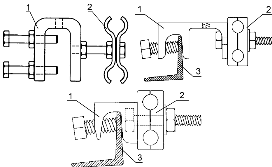
Рисунок 13.10 – Різновиди трубок для закріплення підтримувальних затискачів шлейфового типу: 1 - трубка; 2 - підтримувальний затискач шлейфового типу; 3 - елемент конструкції металевої опори
