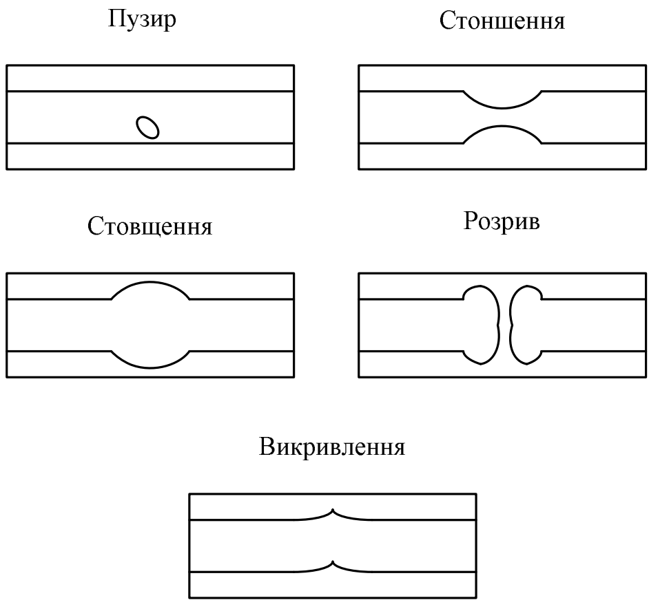
Рисунок 6.14 – Види дефектів при зварюванні ОВ
