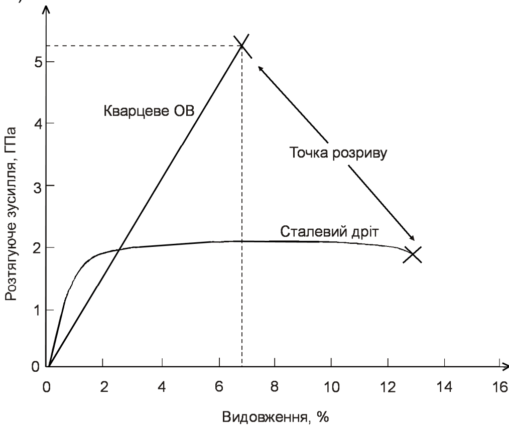
Рисунок 5.41 – Деформація сталевий дроту та ОВ залежно від ступеню розтягу (модуль Юнга: для скла – 72900 \text{ Н/мм}^2 , для сталі – 150000 \text{ Н/мм}^2 )
