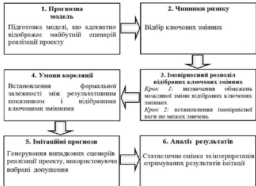
Рис. 1. Блок-схема імітаційного моделювання за методом Монте-Карло
