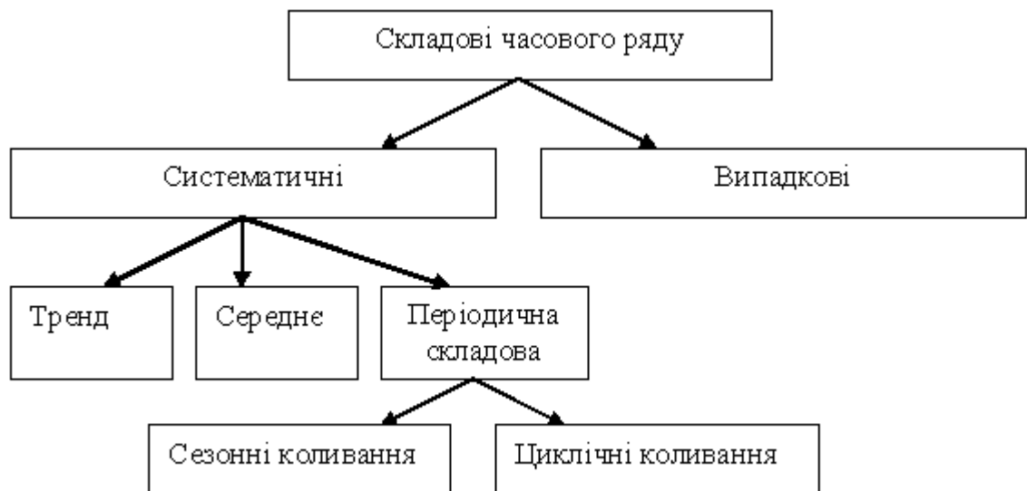
Рис. 2.1. Класифікація складових часового ряду
