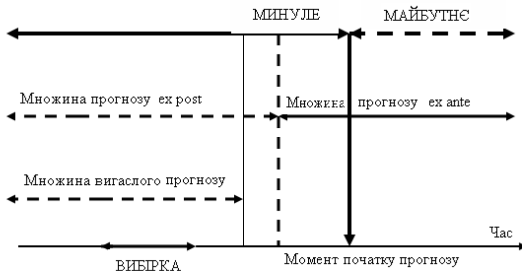
Рис. 1.3. Залежність між прогнозами
