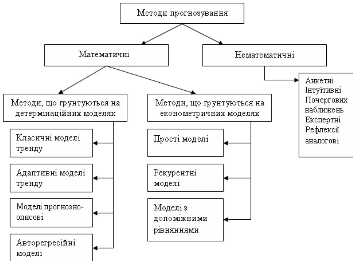
Рис. 1.2. Класифікація методів прогнозування
