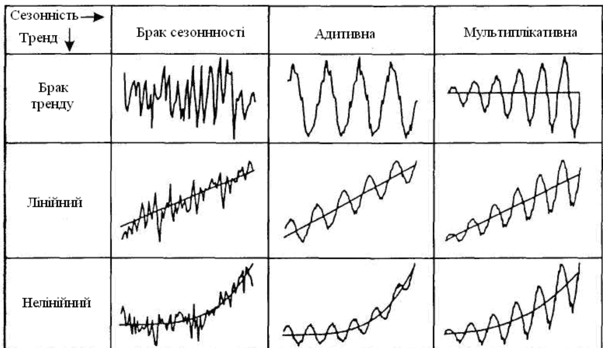
Рис. 2.2. Класифікація часових рядів
