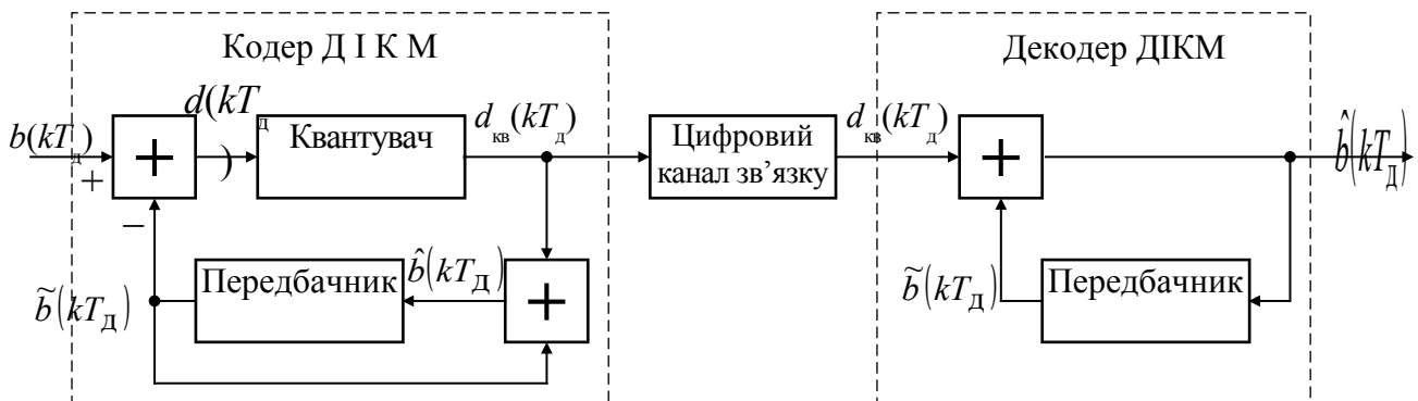
Рисунок 6.2 – Кодер і декодер системи передавання з ДІКМ
