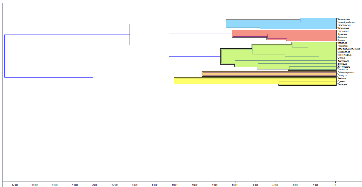
Рис. 2.47. Приклад дендрограми
