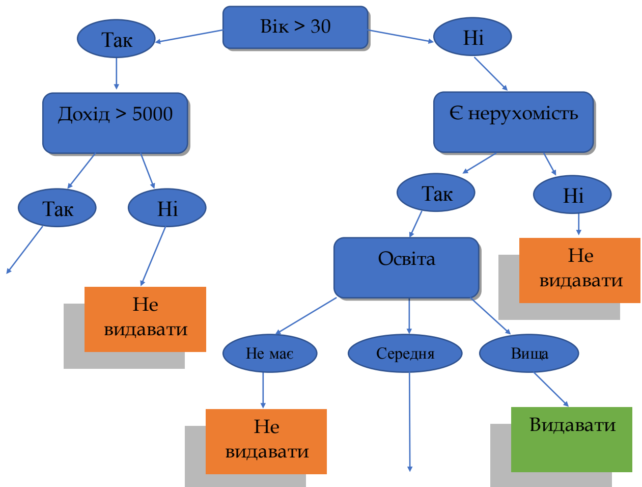
Рис. 3.3. Дерево класифікації
