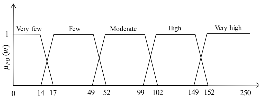
Рис. 2.13. Трапецієвидна функція приналежності для РО
