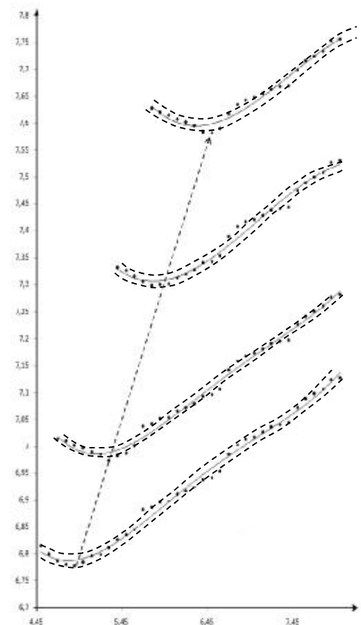
Рис. 2.18б. Дрейф залежності собівартості продукції від інтервалу подачі руди на підприємство при подачі руди різного класу
