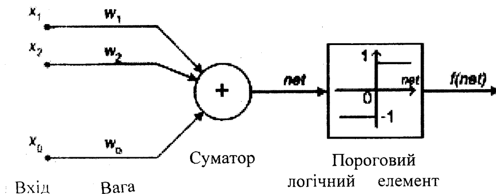
Рис. 2.5. Модель граничного нейрона МакКаллоха-Піттса
