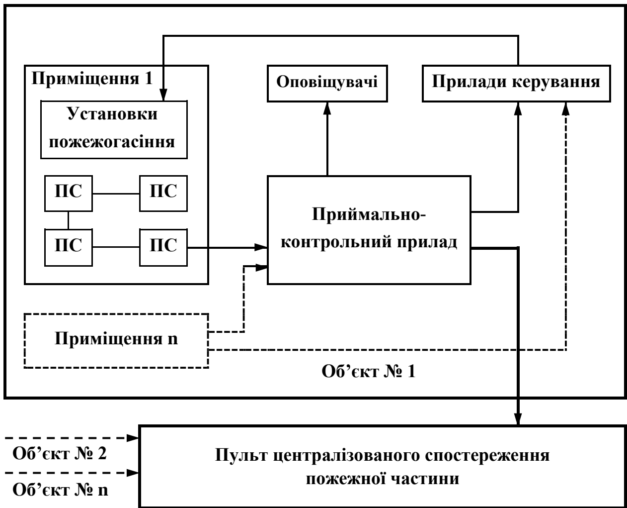
Рис. 2.9. Схема системи пожежної сигналізації (ПС – пожежний сповісник)
